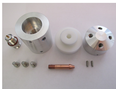
Fig. 3.7 – Antenne démontée. Des tiges en aluminium viennent se glisser dans les filetages présents. [A]
