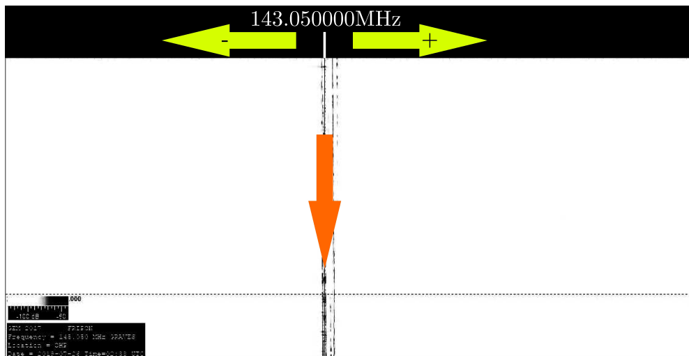
Fig. 3.19 – Les flèches jaunes représentent le décalage Doppler, et la flèche orange le défilement du temps. [A]
