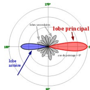
Fig. 2.4 – Coupe horizontale d'un diagramme de rayonnement. [C]
