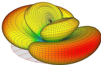
Fig. 2.3 – Exemple de diagramme de rayonnement tridimensionnel. [C]
