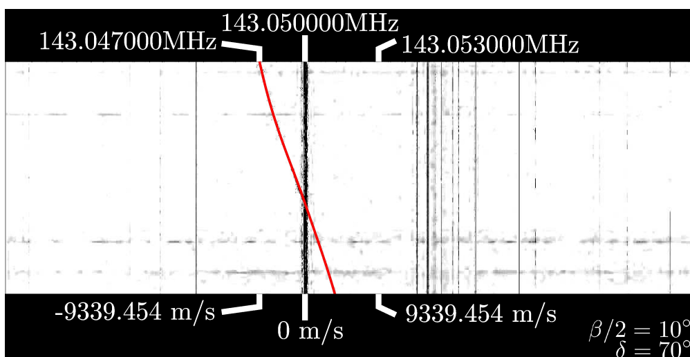
Fig. 5.4 – Détection de l'ISS le 1 juin 2019 à 22h34 [A]
