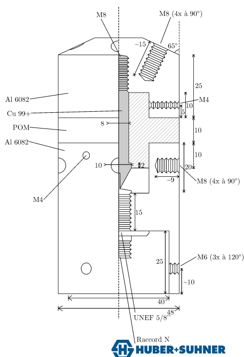
Fig. 3.6 – Schéma de l'antenne mise en place pour effectuer les observations. [A]
