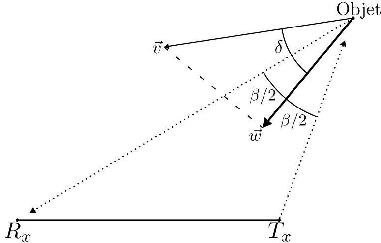
Fig. 2.7 – Représentation géométrique du radar bistatique. [A] Où T_X représente l'émetteur et R_X le récepteur.
