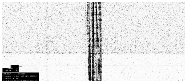
Fig. 5.13 – Parasites obtenus lorsqu'un téléphone portable est placé à côté de l'antenne. [A]
