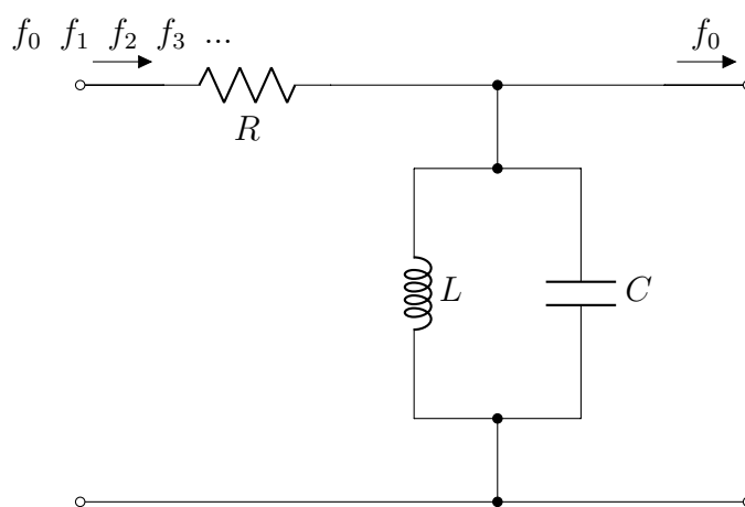
Fig. 3.15 – Exemple de schéma de montage de filtre. Toutes les fréquences sont court-circuitées sauf la fréquence de résonance. [A]
