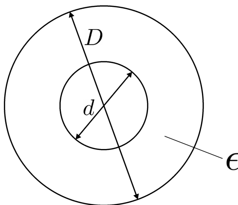
Fig. 2.10 – Coupe verticale d'une ligne coaxiale. [A]
