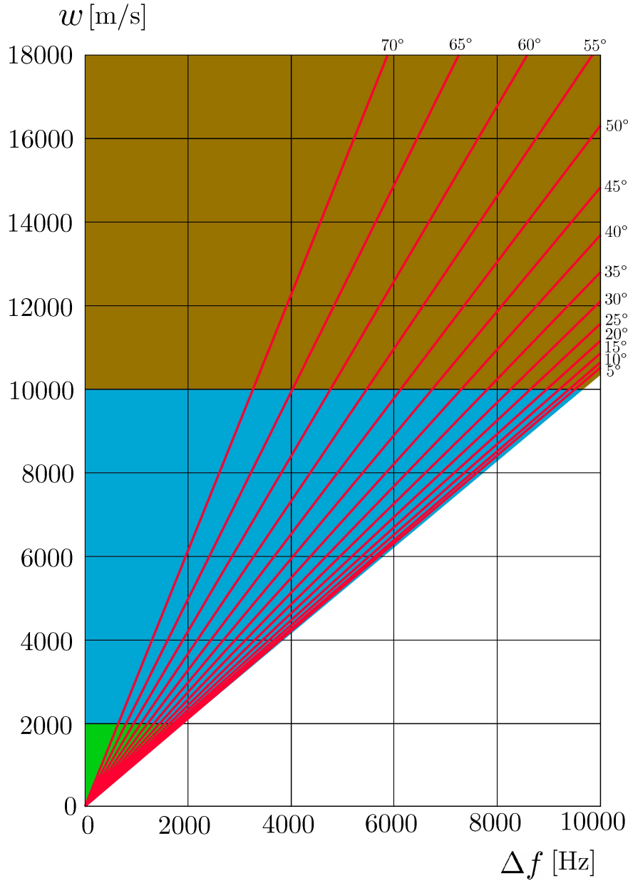
Fig. 2.8 – Abaque représentant la projection de la vitesse en fonction du delta des fréquences et de l'angle bistatique. [A]
