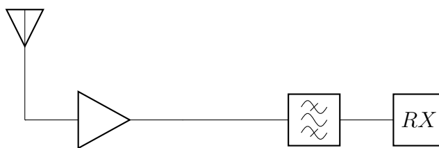
Fig. 3.16 – Schéma de montage comprenant le préamplificateur. [A]
