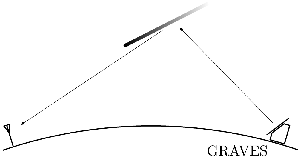
Fig. 2.15 – Fonctionnement général de l'expérience. L'onde est réfléchiée par la traînée occasionnée durant l'ablation. [A]
