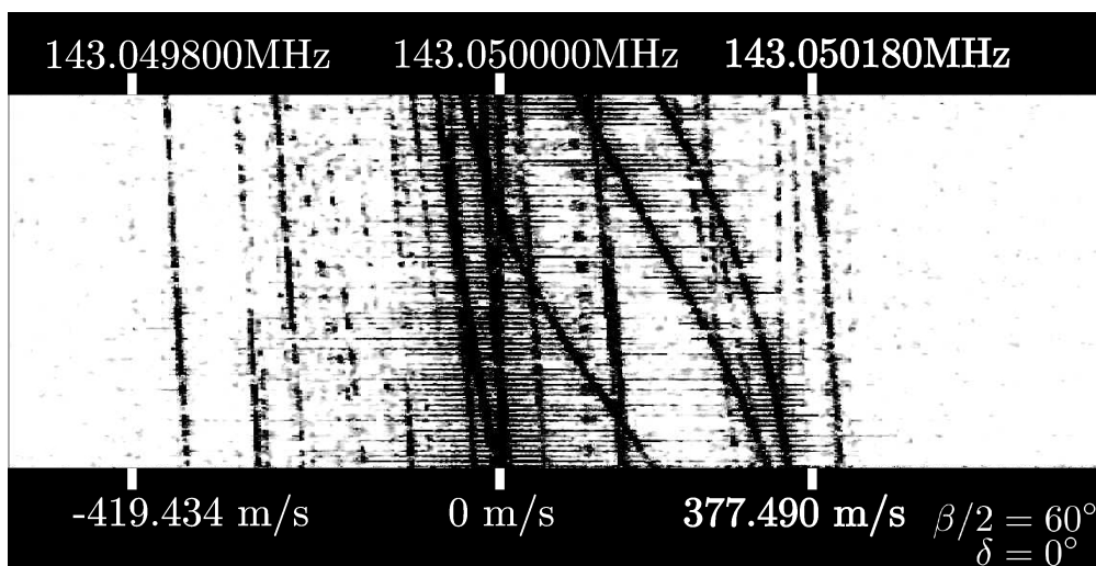
Fig. 5.1 – Signaux obtenu par réflexion contre des avions. [A]
