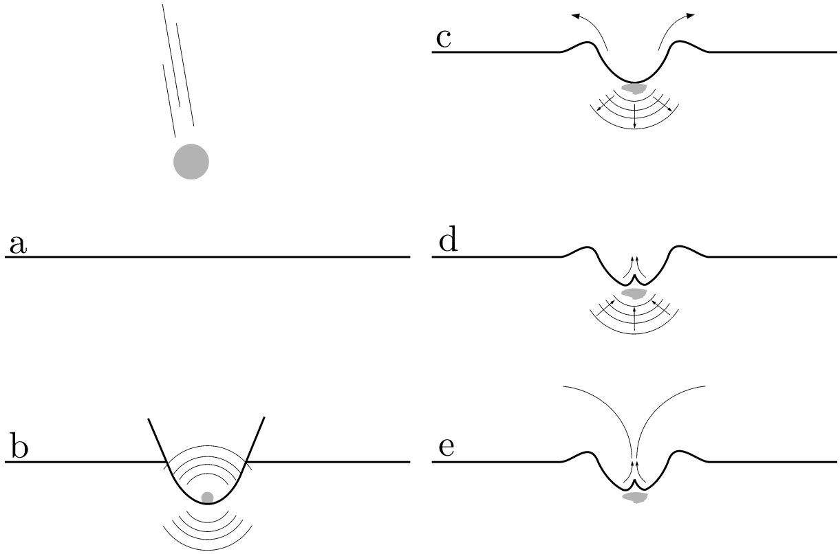
Fig. 2.18 – Différentes phases d'atterrissage d'une météorite. [A]
