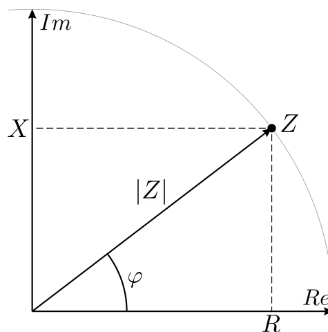
Fig. 2.9 – Représentation graphique de la composante réelle et imaginaire. [A]
