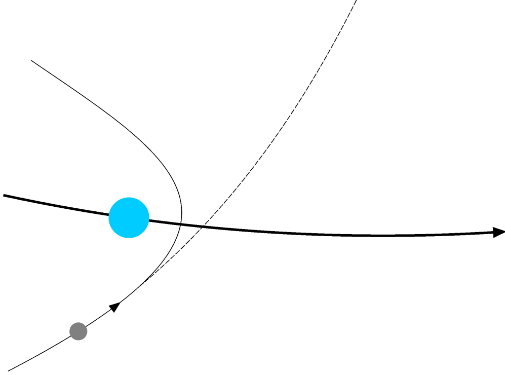
Fig. 2.16 – La terre (disque bleu) dévie l'astéroïde (gris), car ce dernier est entré dans la sphère d'influence de la terre. [A]
