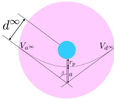
Fig. 2.17 – Représentation de la sphère d'influence d'un corps (par exemple la terre). [A]
