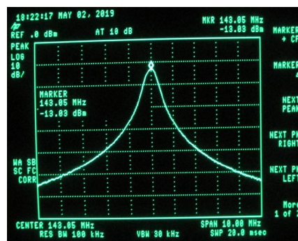
Fig. 3.14 – Analyse spectrale de la seconde cavité (filtre gris sur la Fig. 3.12). [A]
