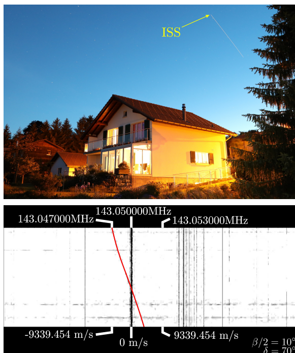
Figure 10 – Deux illustrations de l’ISS enregistrées simultanément : optiquement (photographie) et par détection radar bistatique.
