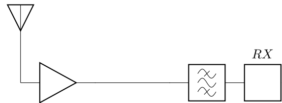
Figure 5 – Schéma bloc du système de réception placé sur le toit de la Halle de gymnastique du Gymnase des Alpes de Bienne.
